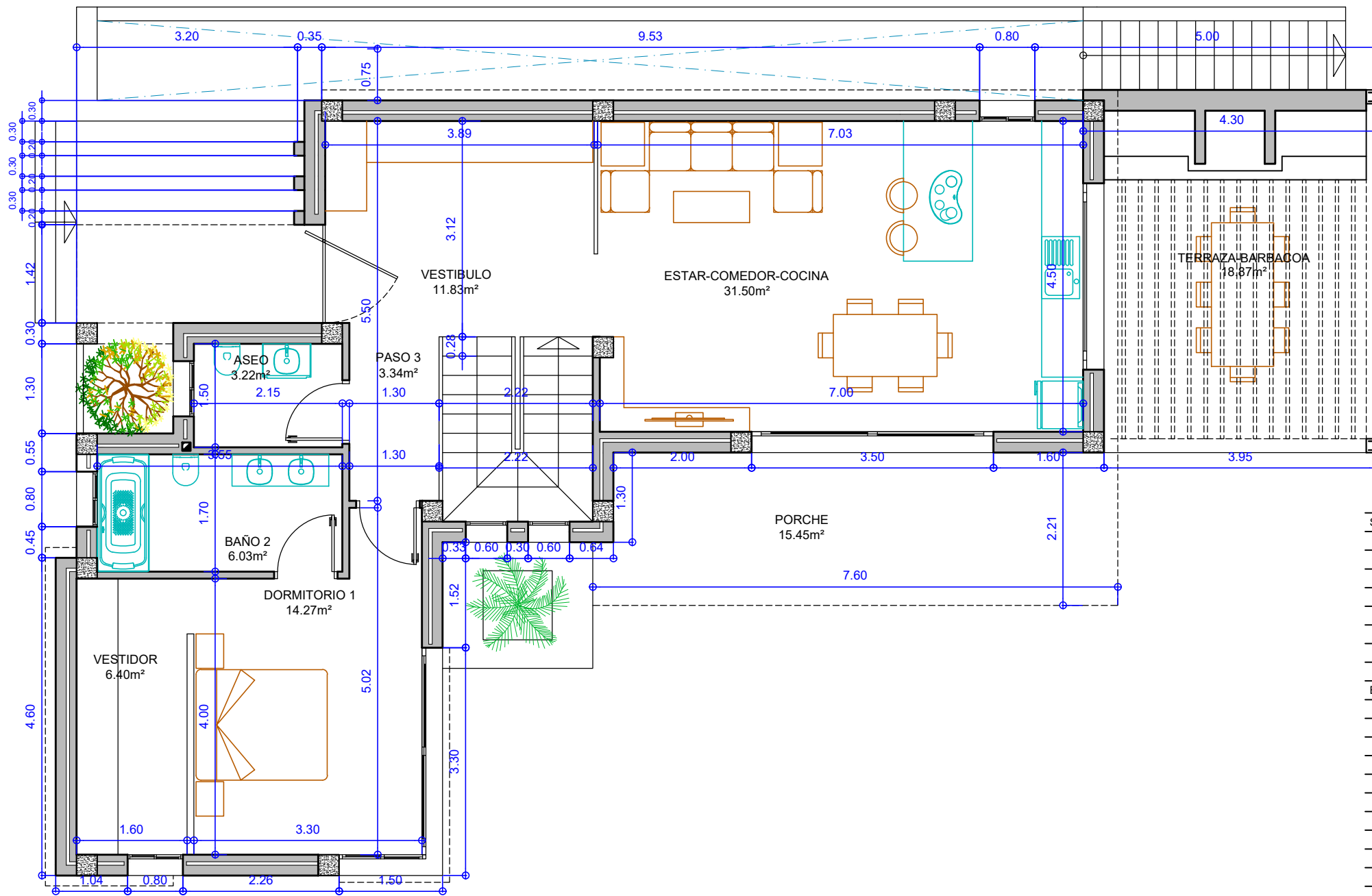
PLANTA BAJA
